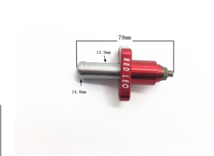
JY-4731 涨紧器
