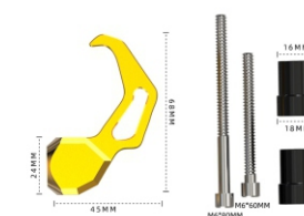
尺寸参数
